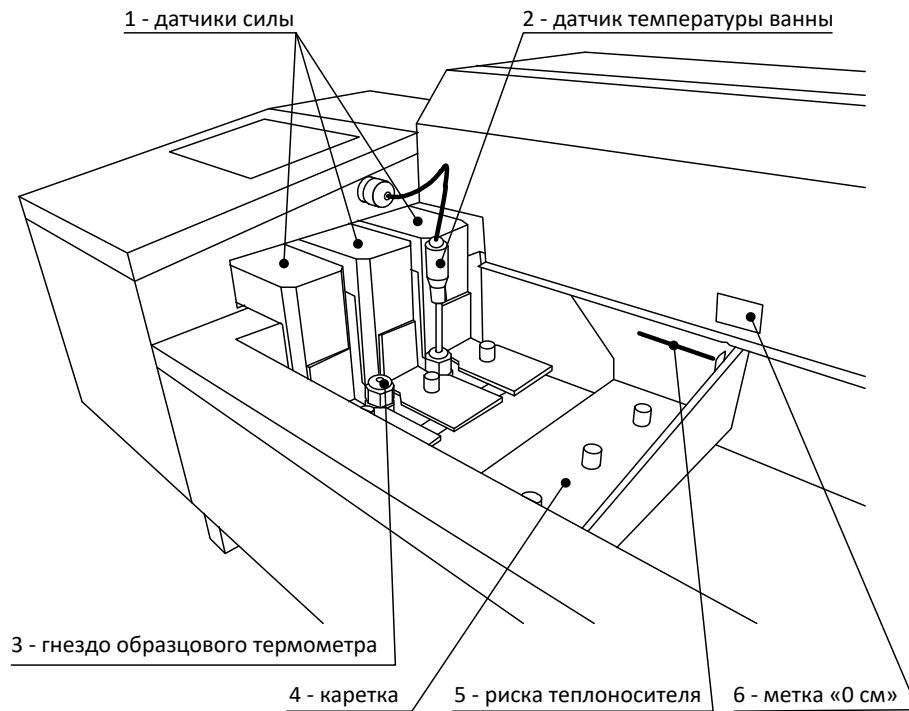
Рисунок 4– Система нагружения
