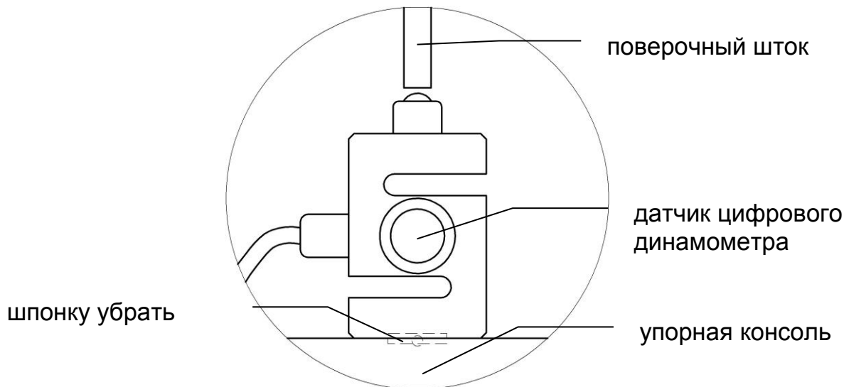
Рисунок 2 – Установка датчика электронного динамометра
