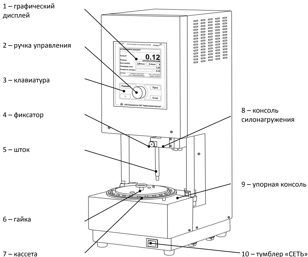
Рисунок 1 – Общий вид прочномера
